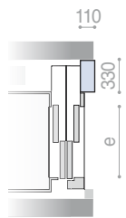
Poziționare panou mentenanță
