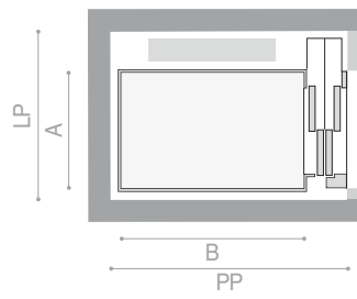
Plan un singur acces
