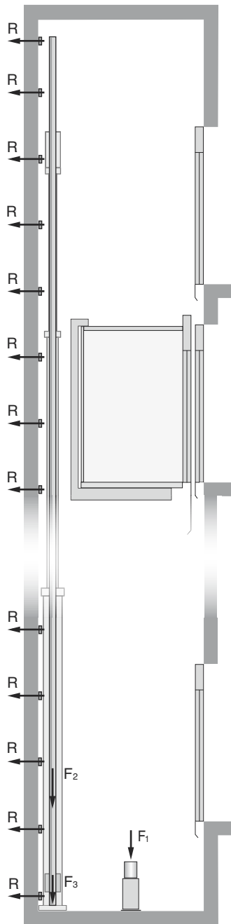
Elevație (piston spate)
