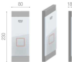
Panou operare și control palier Cod: SPW 7
