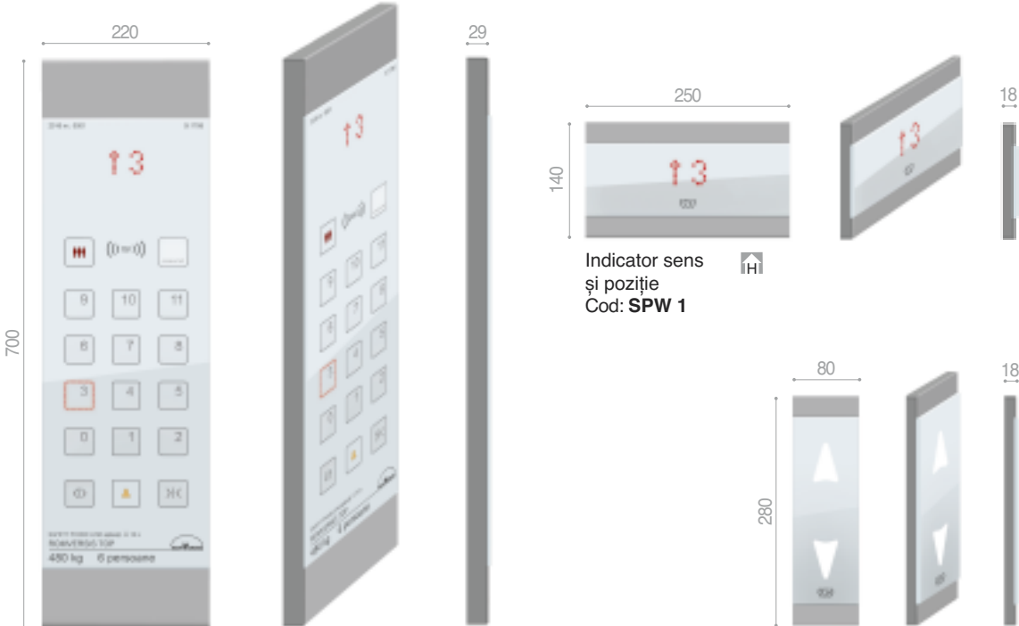
Panou operare și control cabină Cod: PSPW 1
